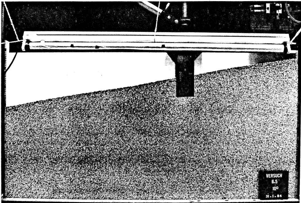
Abb. 1: Versuchsaufbau: Schneebeli-Modell mit Aluminiumstäbchen, Fundament und hydraulischer Pumpe; im Vordergrund ist eine UV-Leuchtstoffröhre aufgehängt. Aufnahme bei Tageslicht: Die Stäbchen bilden sich als gleichförmige Masse ab. (Ausschnitt, M=1:12)
